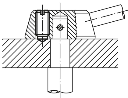
Фиксатор рукоятки
